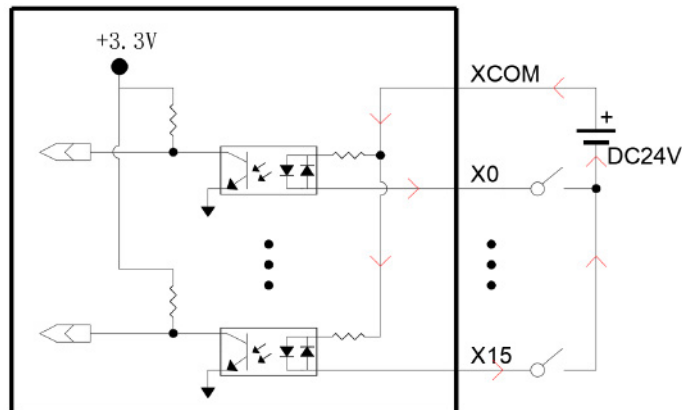
Figure 6 DI NPN wiring solution
