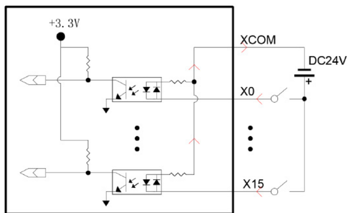
Figure 7 DI PNP wiring solution
